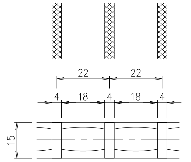
メインバーピッチ詳細図 S=1/1
