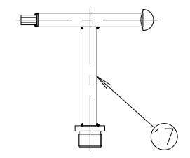
ハンドル (MF-44) S=1/5
