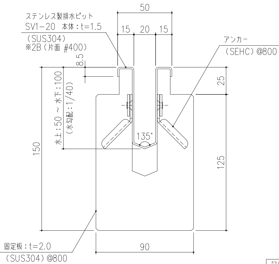
ピット断面詳細図 S=1/2
