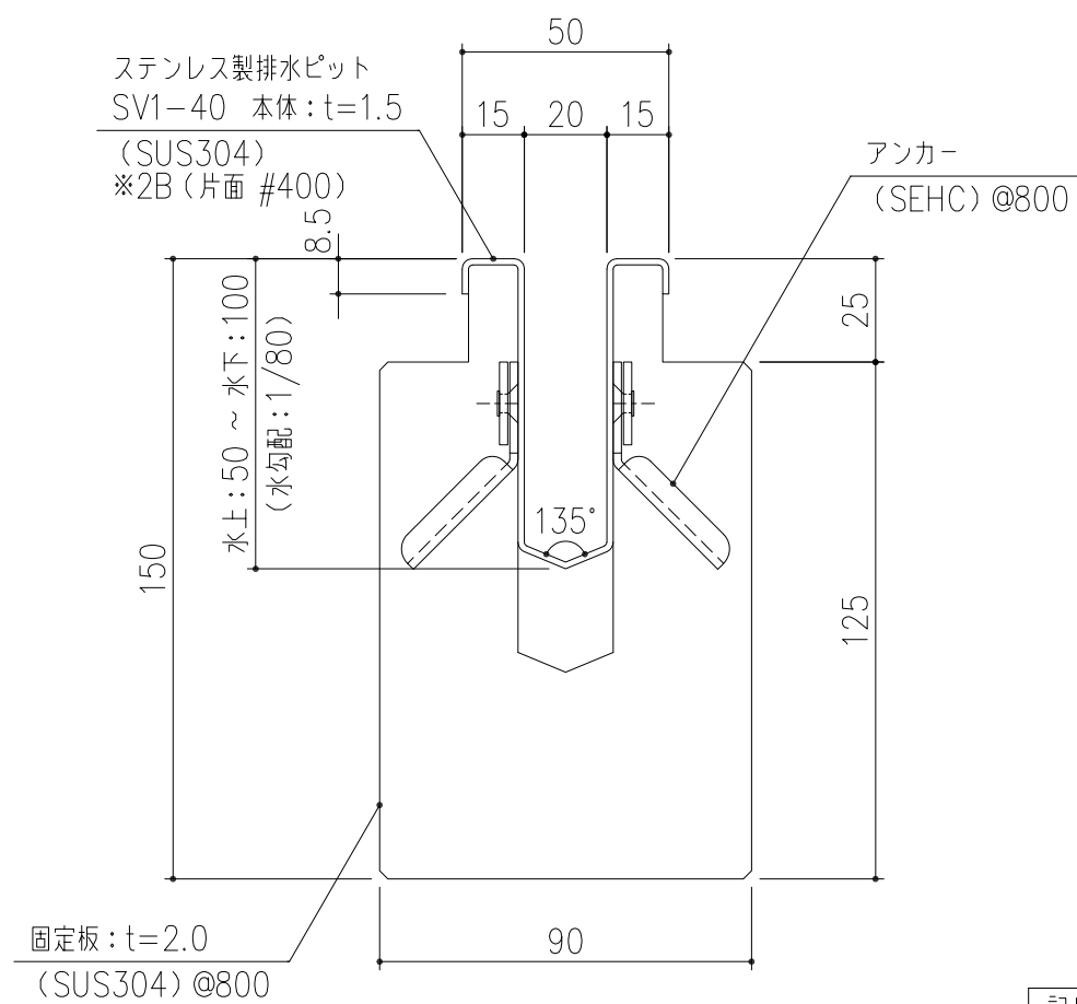
ピット断面詳細図 S=1/2
