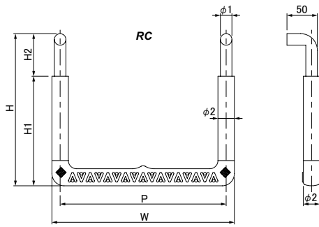
●寸法表 芯材:SWCH12R(芯材:SUS304)
