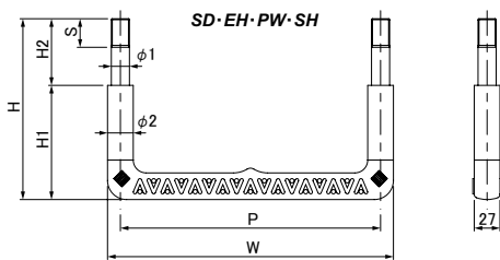
●寸法表(芯材:SWCH12R)
