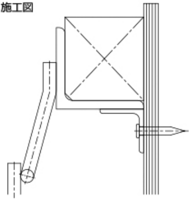
施工図
