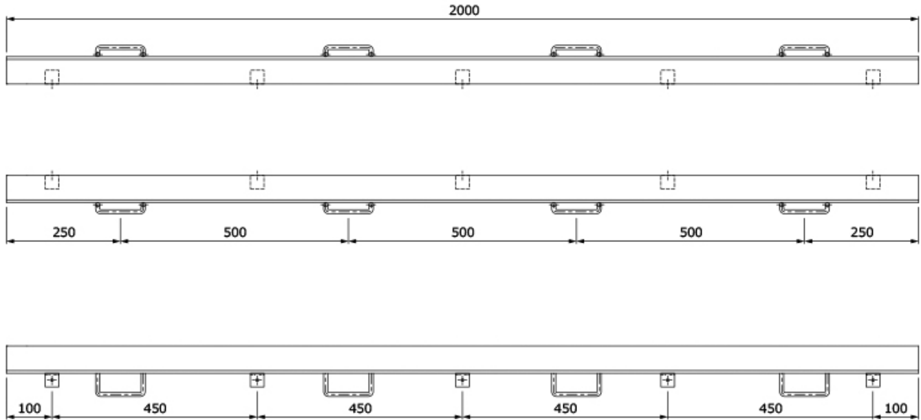
受枠断面図
