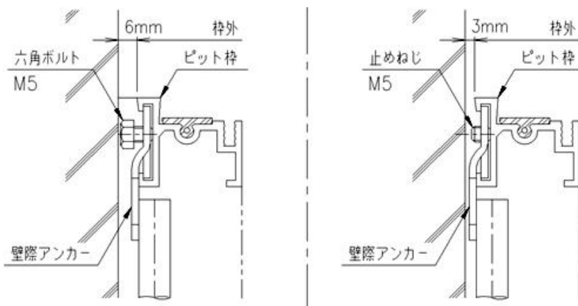
断面納まり図
