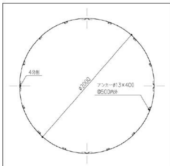
平面図 (参考)
