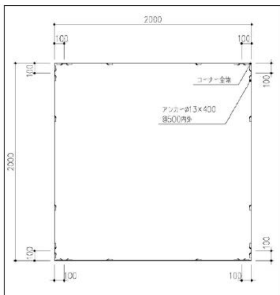
平面図 (参考)
