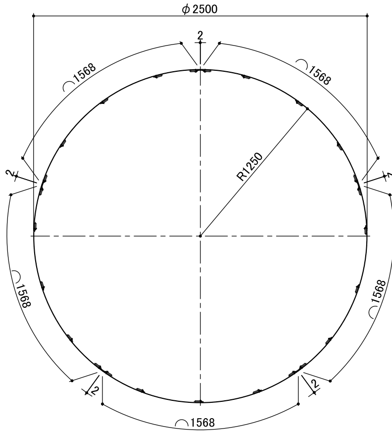
平面図(参考)
