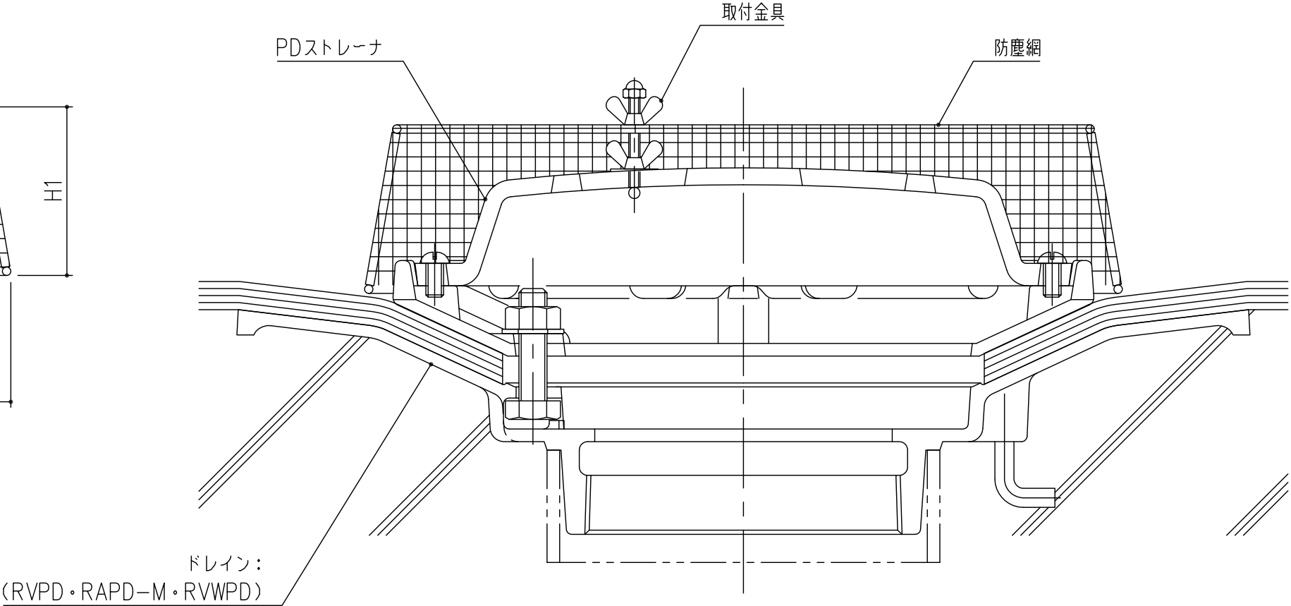
施工例
