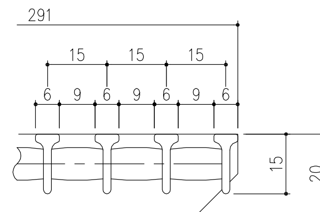
メンバー端部詳細図 S=1/1
