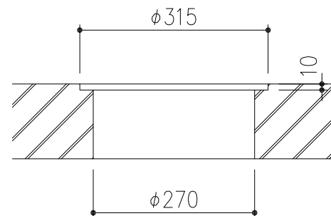
取付孔寸法
