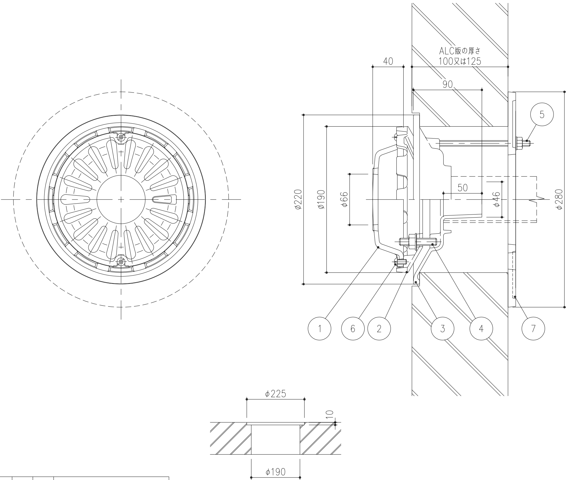
取付孔寸法
