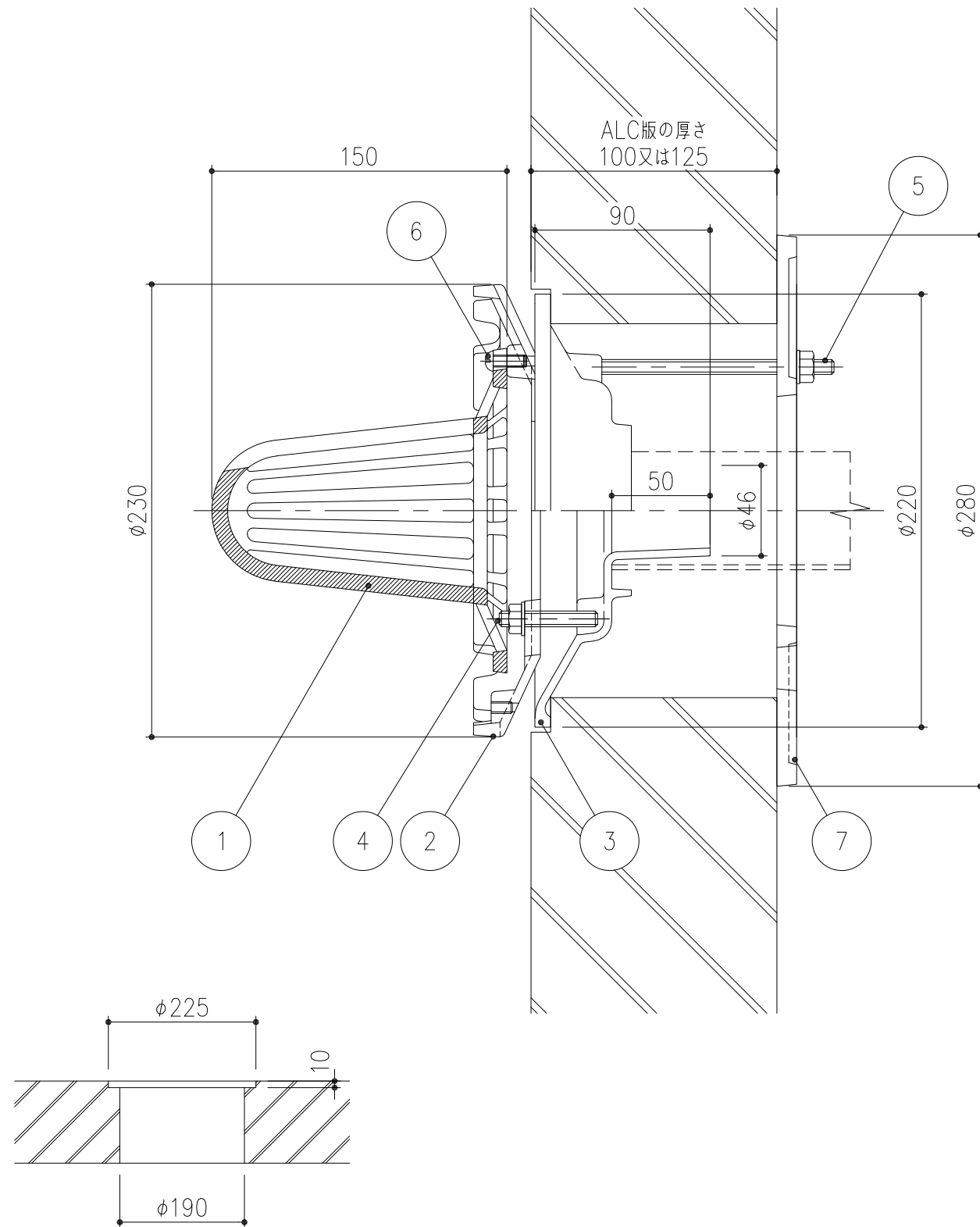
取付孔寸法
