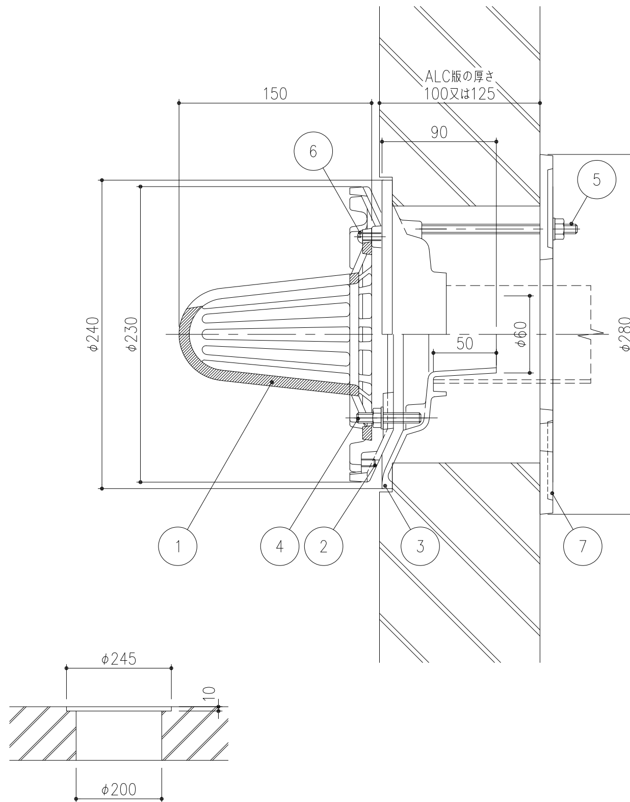
取付孔寸法
