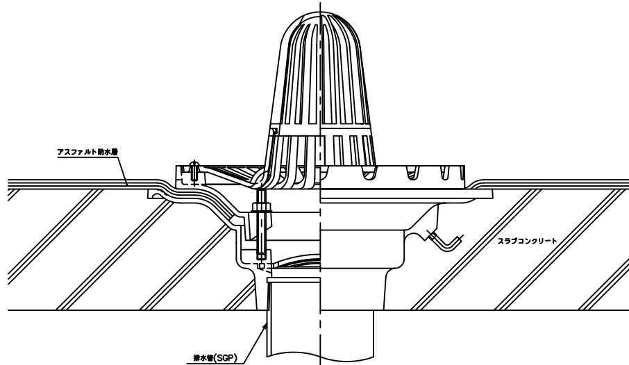
アスファルト露出防水
