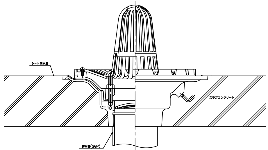
シート露出防水
