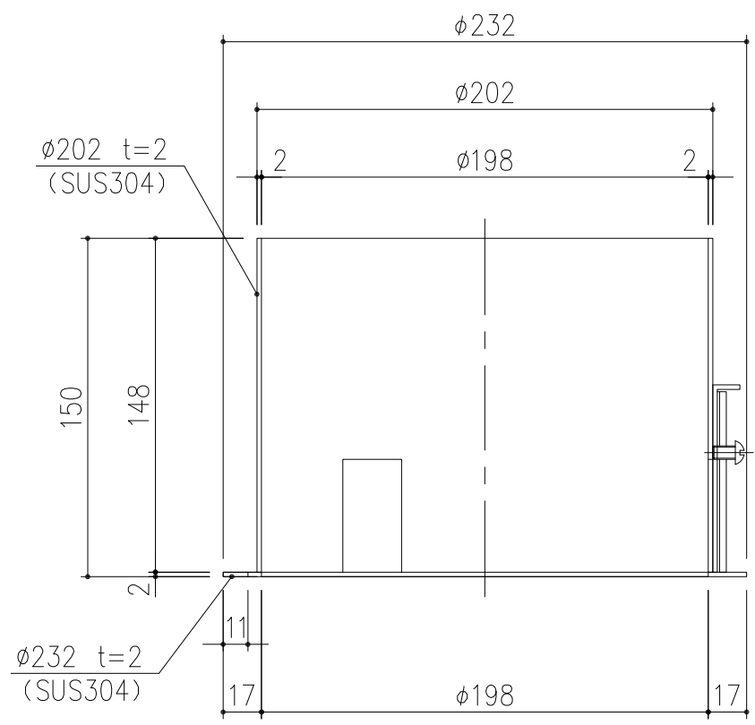
雨量調整金物 詳細図
