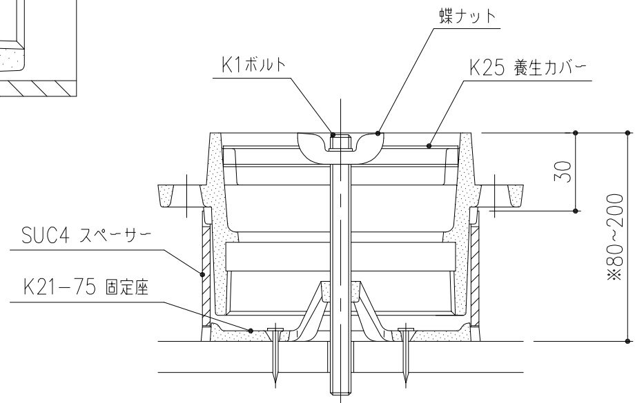
打込金具セット状態図 S=1/2
