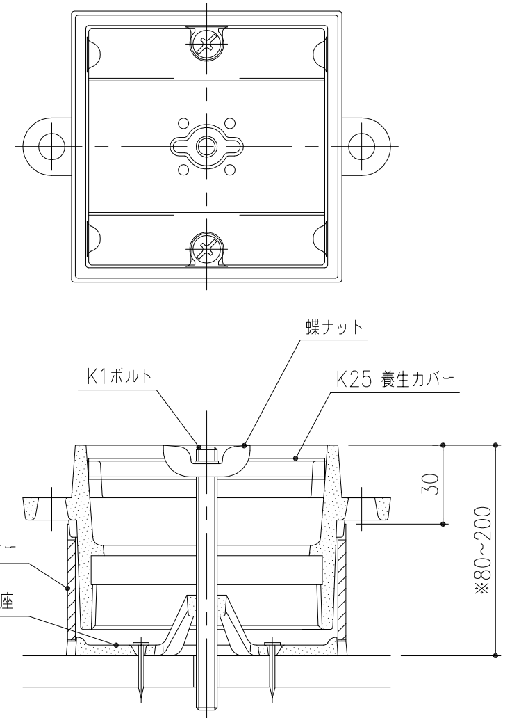
打込金具セット状態図 S=1/2
