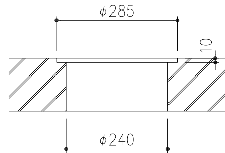
取付孔寸法
