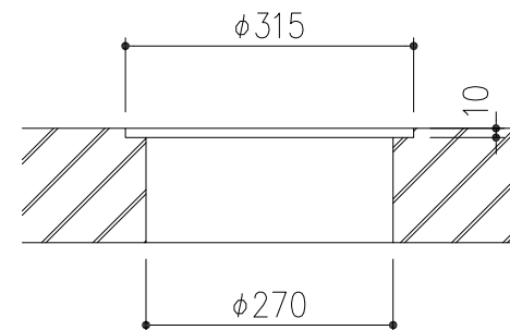
取付孔寸法
