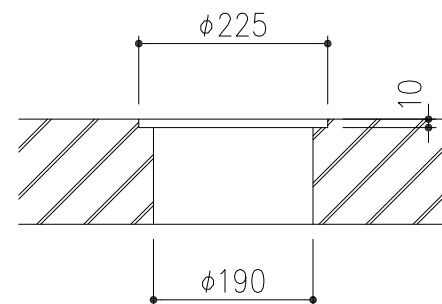
取付孔寸法
