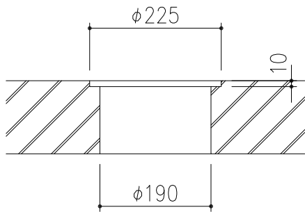
取付孔寸法
