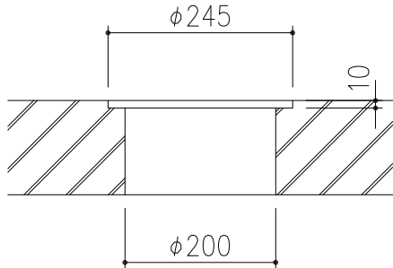
取付孔寸法
