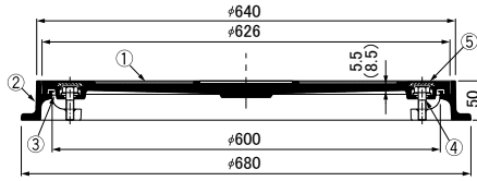
( )寸法 = MCA-RL シリーズ
