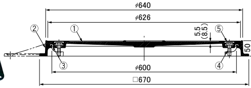
( )寸法 = MCA-L シリーズ
