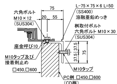
柵取付金具部拡大図
