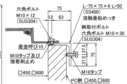
柵取付金具部拡大図
