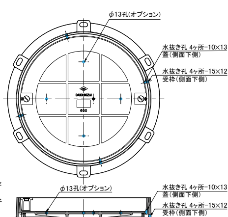
化粧蓋・丸形(例:MIB-R2シリーズ)
