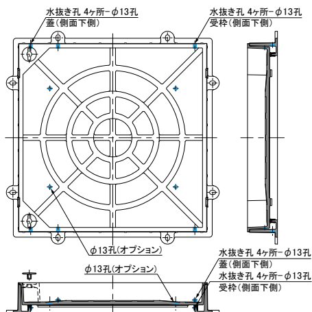
化粧蓋・角形(例:MHIBシリーズ)
