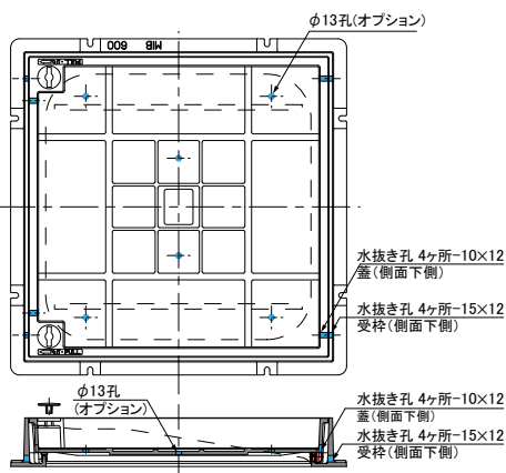
化粧蓋・角形(例:MIBシリーズ)
