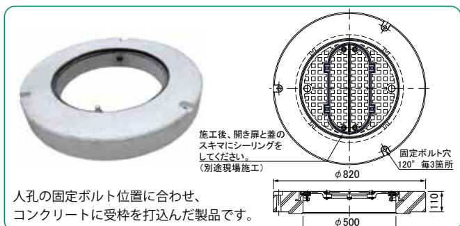
MEWC 一体型台座（人孔用）
