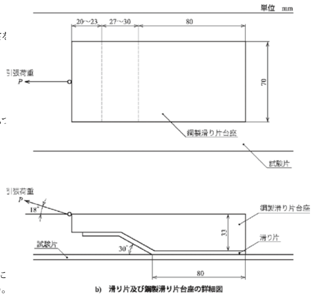
図11—滑り試験機（続き）
