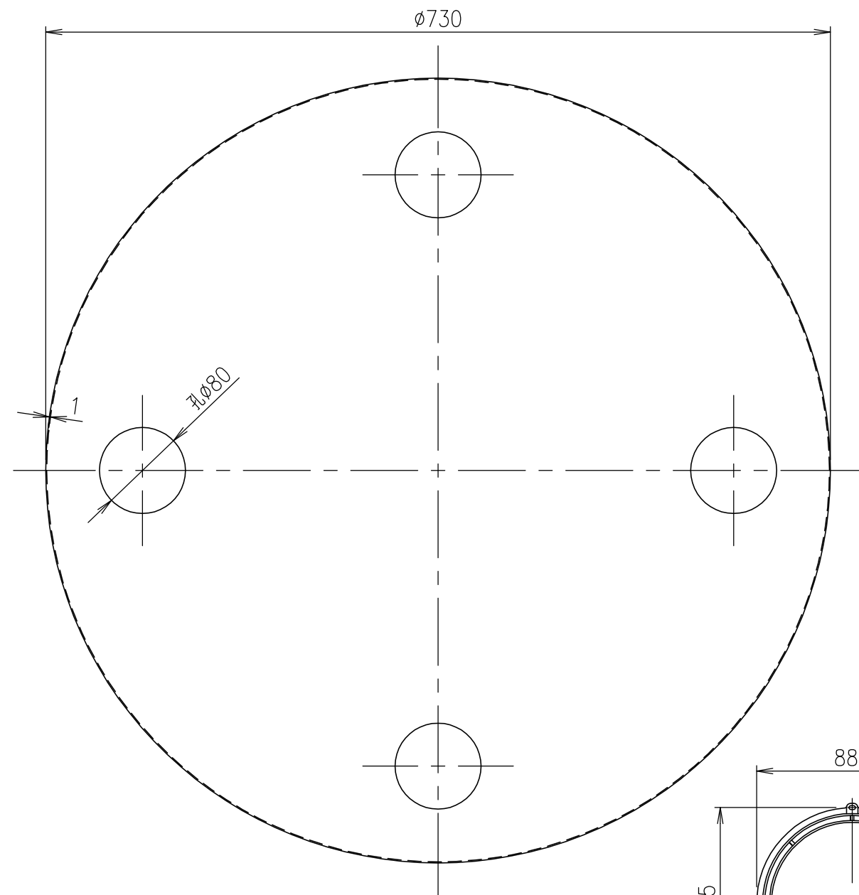
断熱保護カバー詳細図
