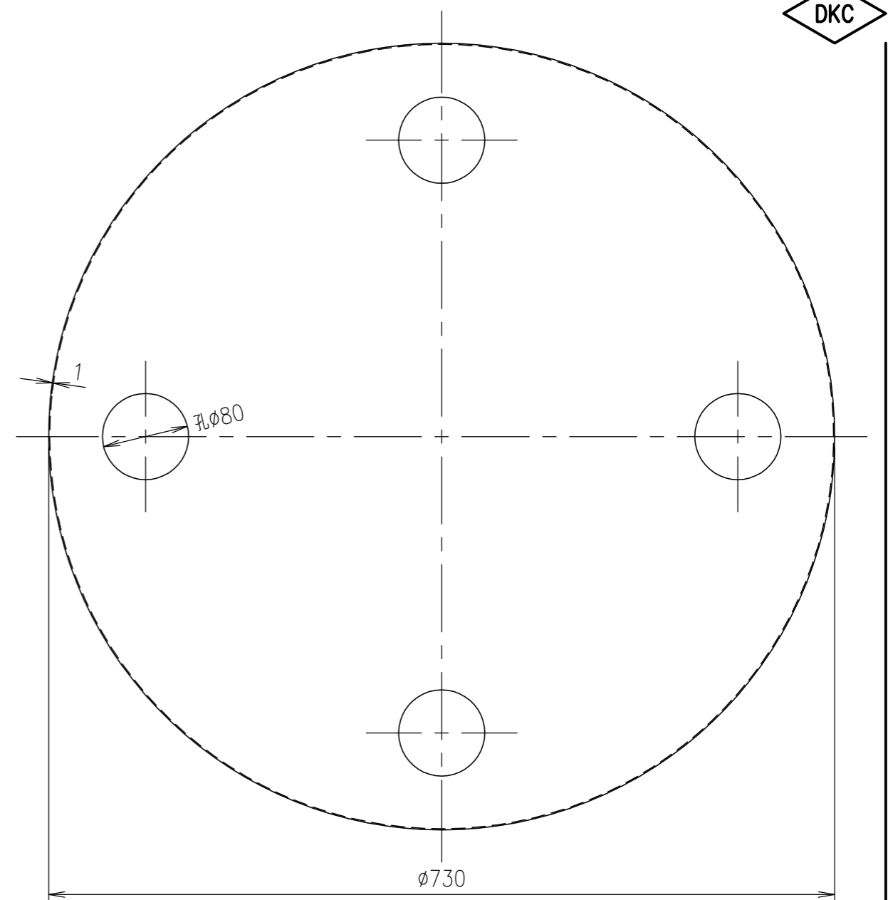
断熱保護カバー詳細図
