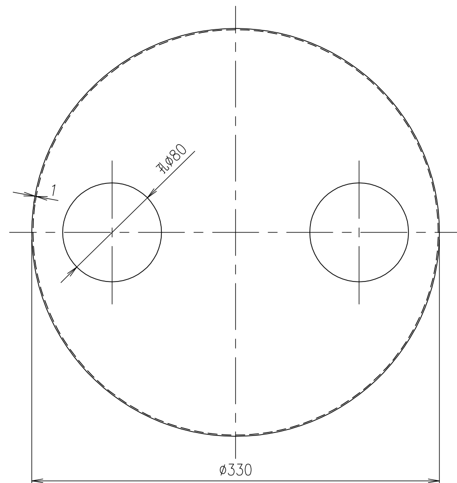
断熱保護カバー詳細図
