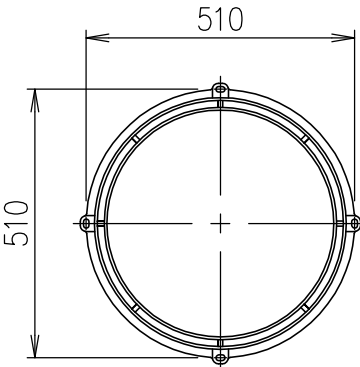
アンカーボルト位置寸法
