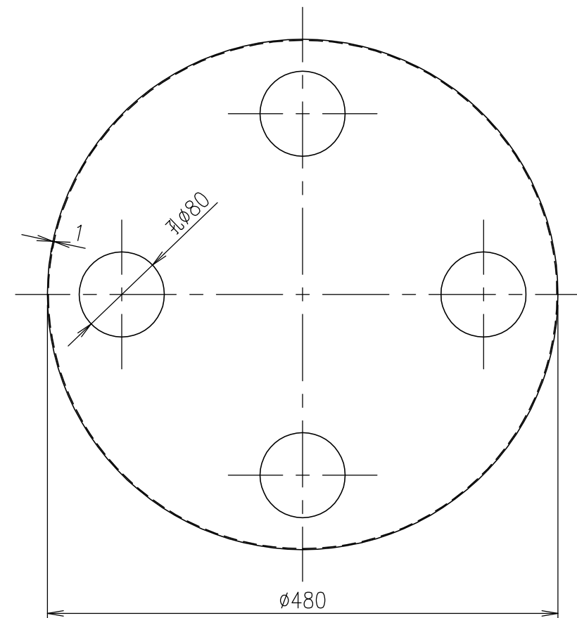
断熱保護カバー詳細図
