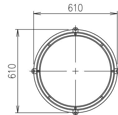
アンカーボルト位置寸法
