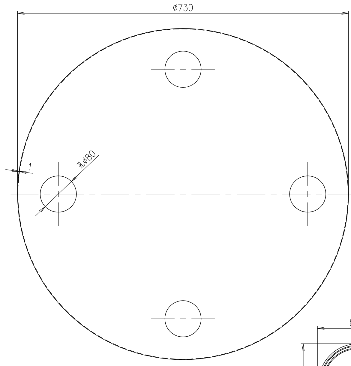
断熱保護カバー詳細図
