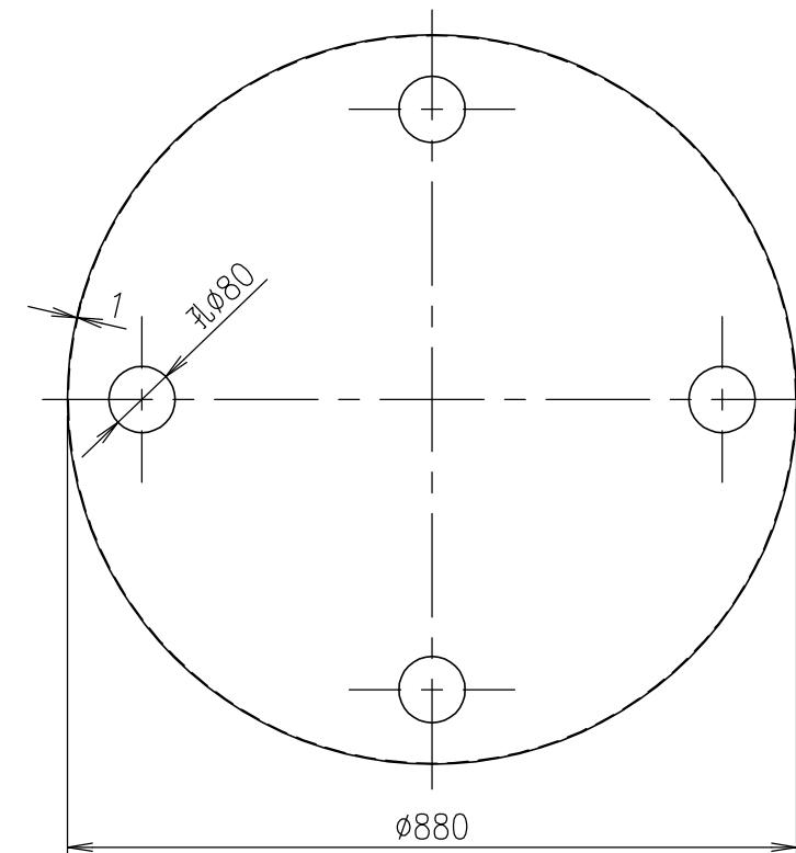
断熱保護カバー詳細図
