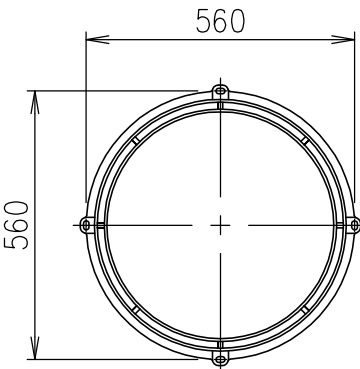
アンカーボルト位置寸法
