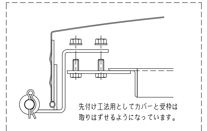
施工参考図
