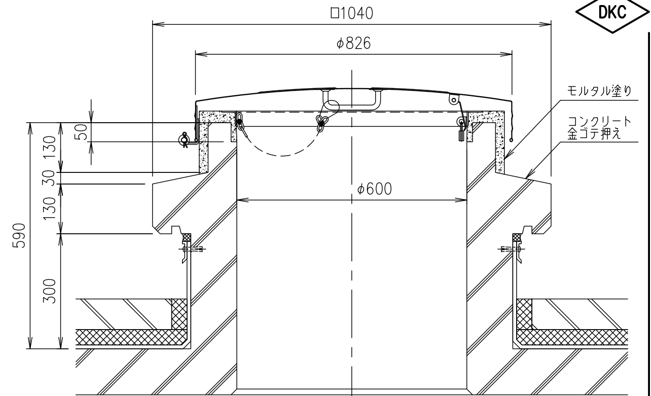
施工参考図
