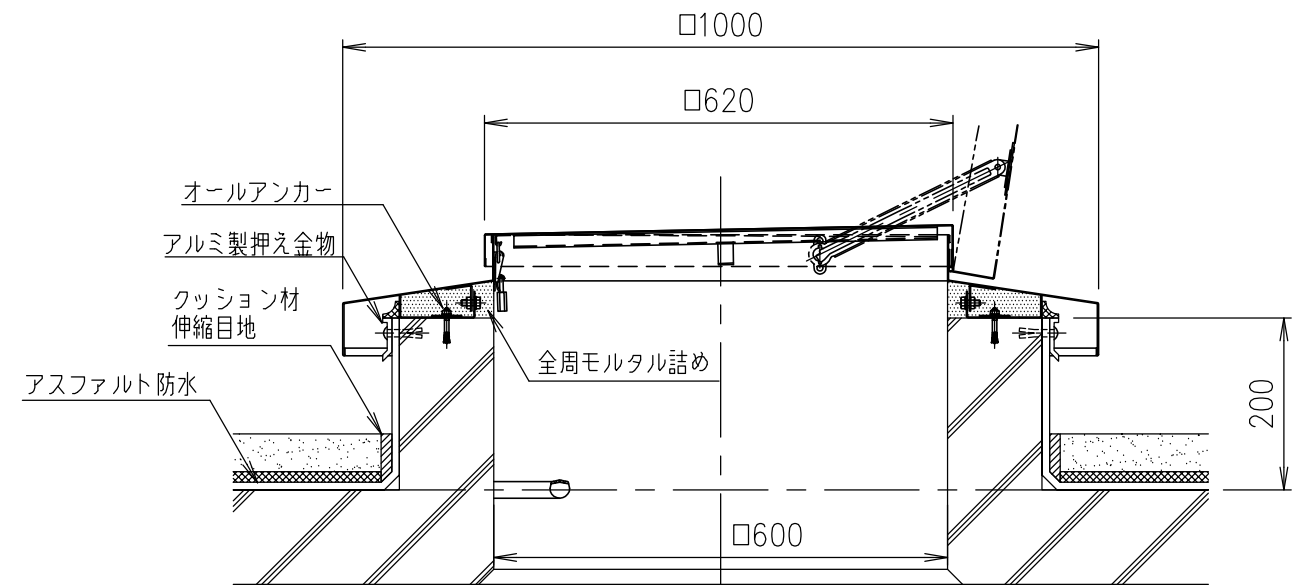
施工参考図
