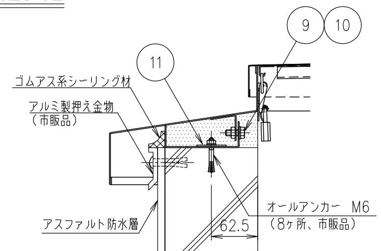
部分詳細図 S=1/5
