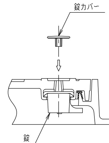
錠部断面図 S=1/5
