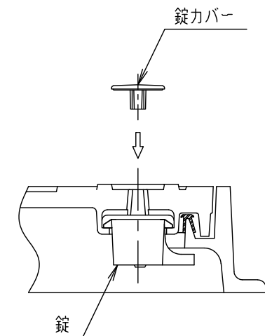
錠部断面図 S=1/5
