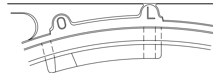
ロック部詳細図 S=1/2
