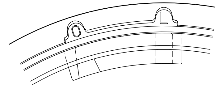
□ツク部詳細図 S=1/2
