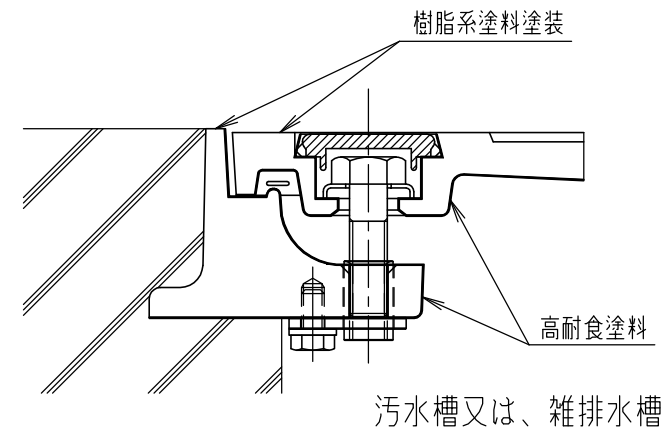
A-A断面詳細図 S=1/2
