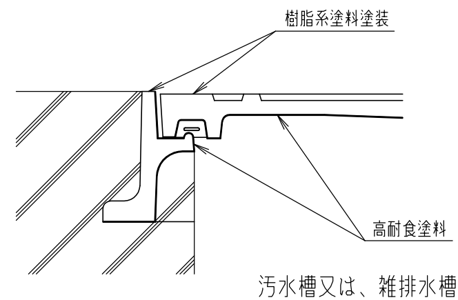
B-B断面詳細図 S=1/2
