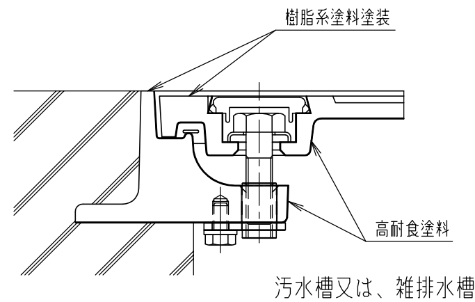
A-A断面詳細図 S=1/2
