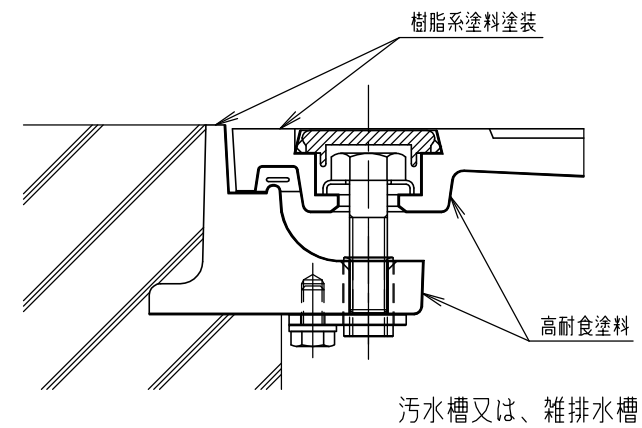
A-A断面詳細図 S=1/2
