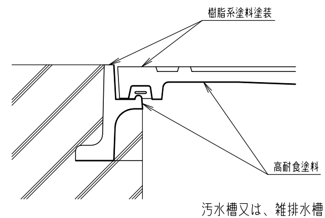
B-B断面詳細図 S=1/2
