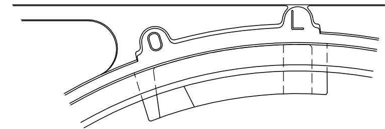
□ツク部詳細図 S=1/2
