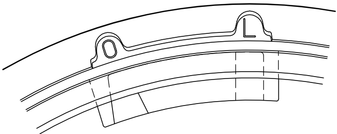
ロック部詳細図 S=1/2
