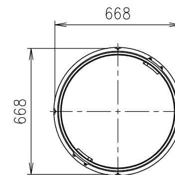
アンカーボルト位置寸法
