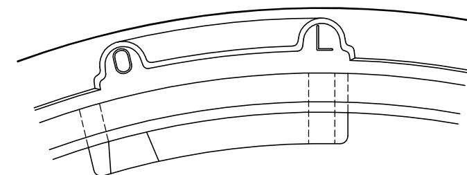
ロック部詳細図 S=1/2
