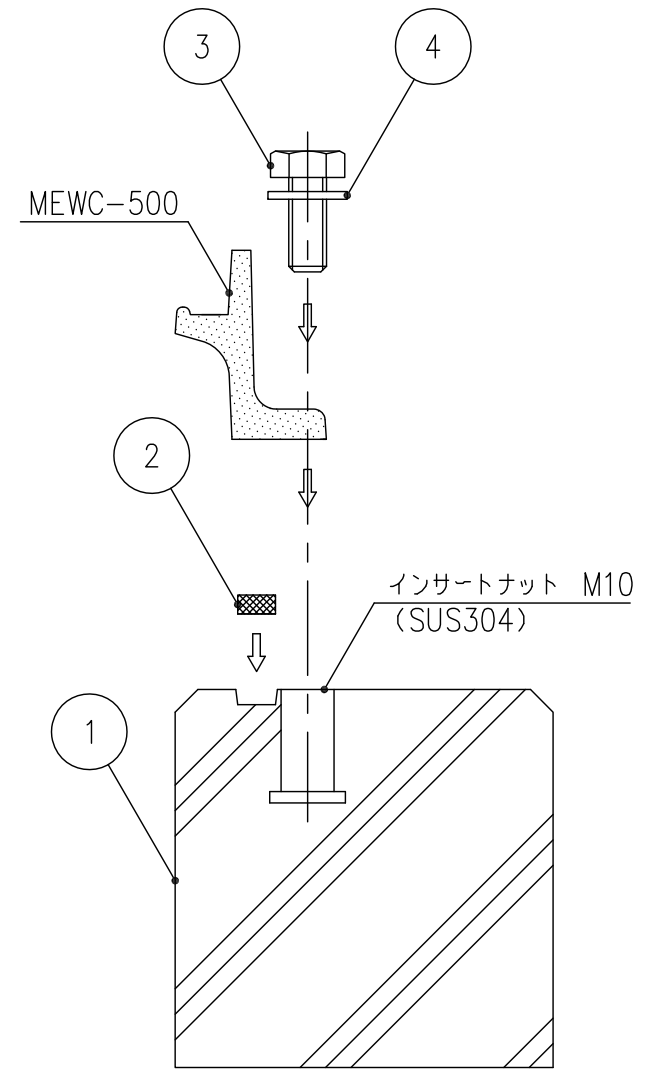
組立手順図 S=1/2
